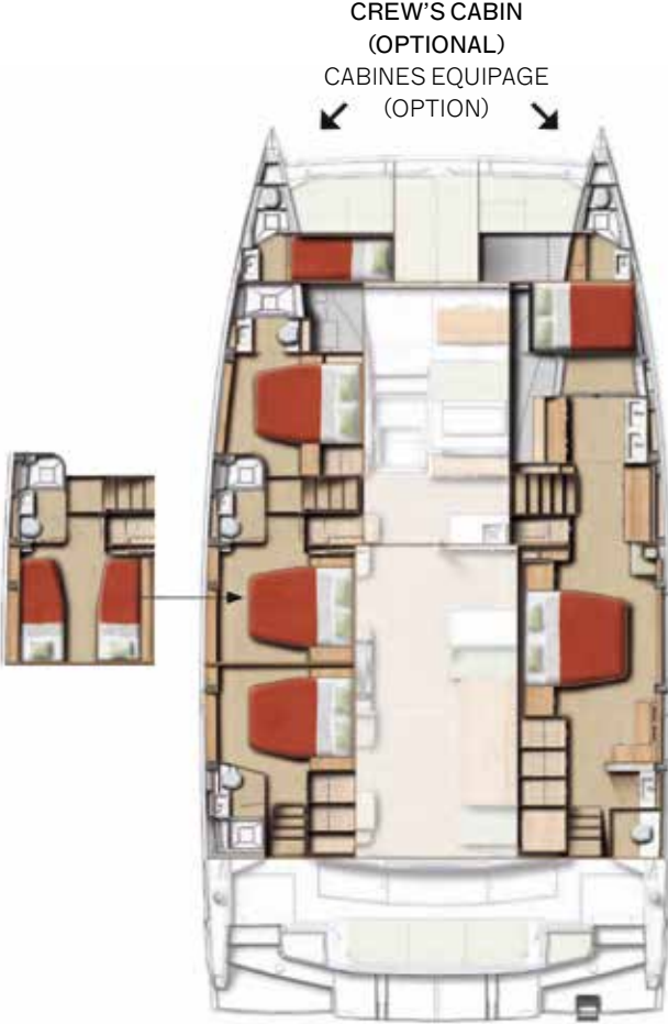
4 DOUBLE CABINS (OWNER'S VERSION) / 4 BATHS Version 4 cabines doubles (propriétaire) / 4 sdb
